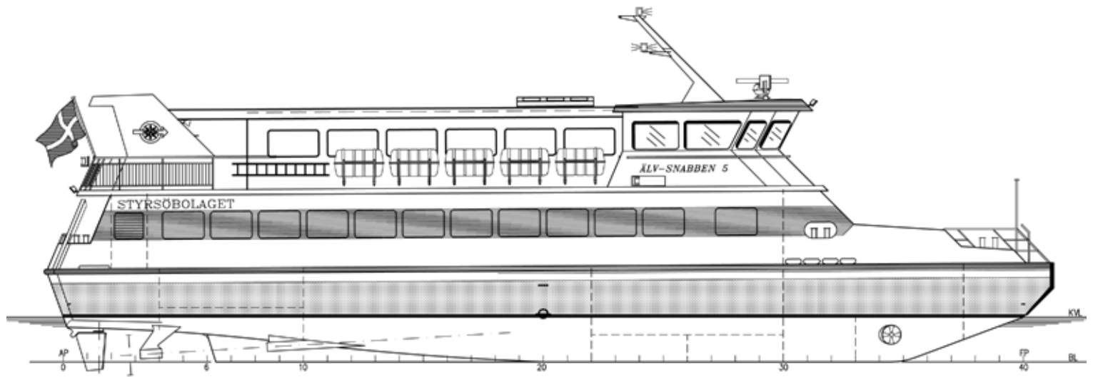
SIDOVY
